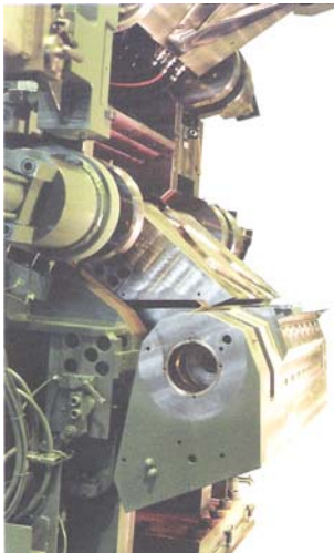
液压开合 液压口型锁紧 四复合机头
